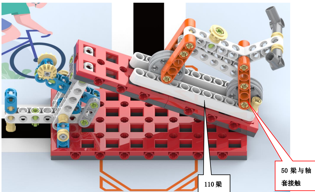
图 7 完成状态
